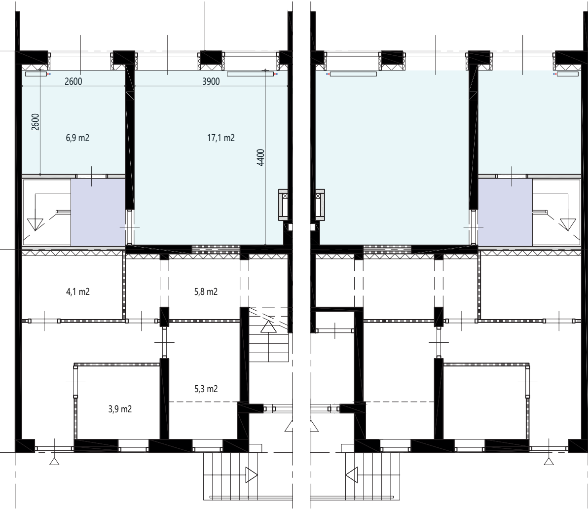
Begane grond
